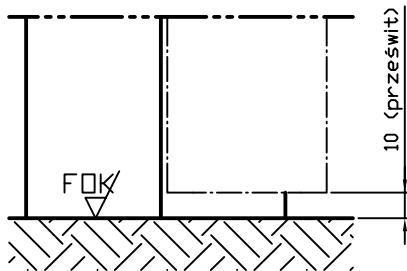
Bez progu Min. Wmurowanie w posadzce: bez
