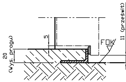
Próg z kątownikiem (20) Skrzydło z felcem w dolnej części Min. Wmurowanie w posadzce: Bez
