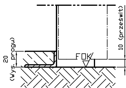
próg z kątownikiem (20 mm) Min. Wmurowanie w posadzce: bez
