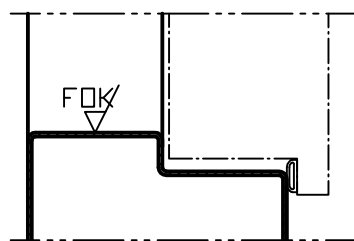
Osłonecznica obwiedniowa Skrzydło z felcem w dolnej części
