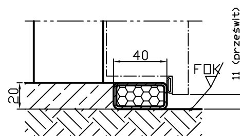
Próg z rury kwadratowej (20) Skrzydło z felcem w dolnej części Min. Wmurowanie w posadzce: Bez
