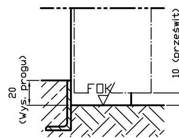
próg z kątownikiem (40 mm) Min. Wmurowanie w posadzce: 20 mm
