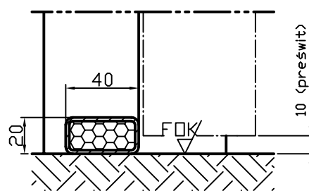
próg z rury kwadratowej (20 mm) Min. Wmurowanie w posadzce: bez
