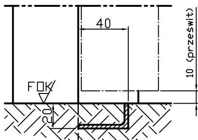
Szyna dzieląca (20 mm) Min. Wmurowanie w posadzce: 20 mm
