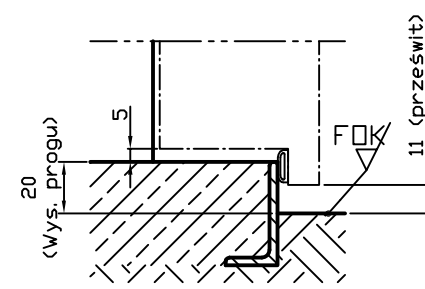
Próg z kątownikiem (40 mm) Skrzydło z felcem w dolnej części Min. Wmurowanie w posadzce: 20 mm
