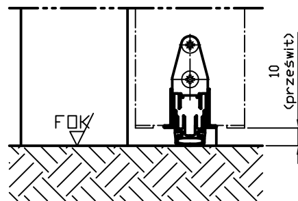
Uszczelka podłogowa opadająca Planet PU
